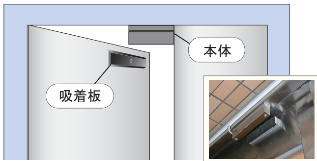
側面取付金具を使用する場合
