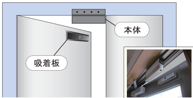
L 型 or BOX 型取付金具を使用する場合
